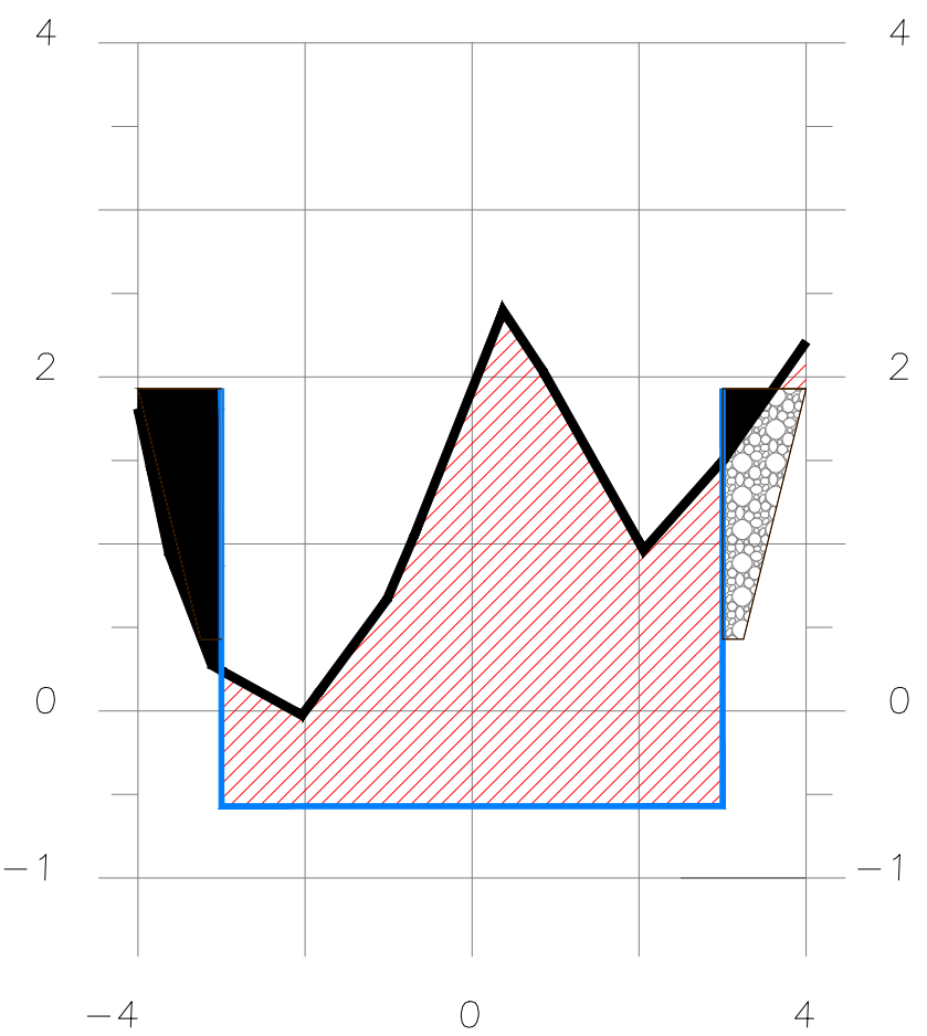
SECCION 3+090
