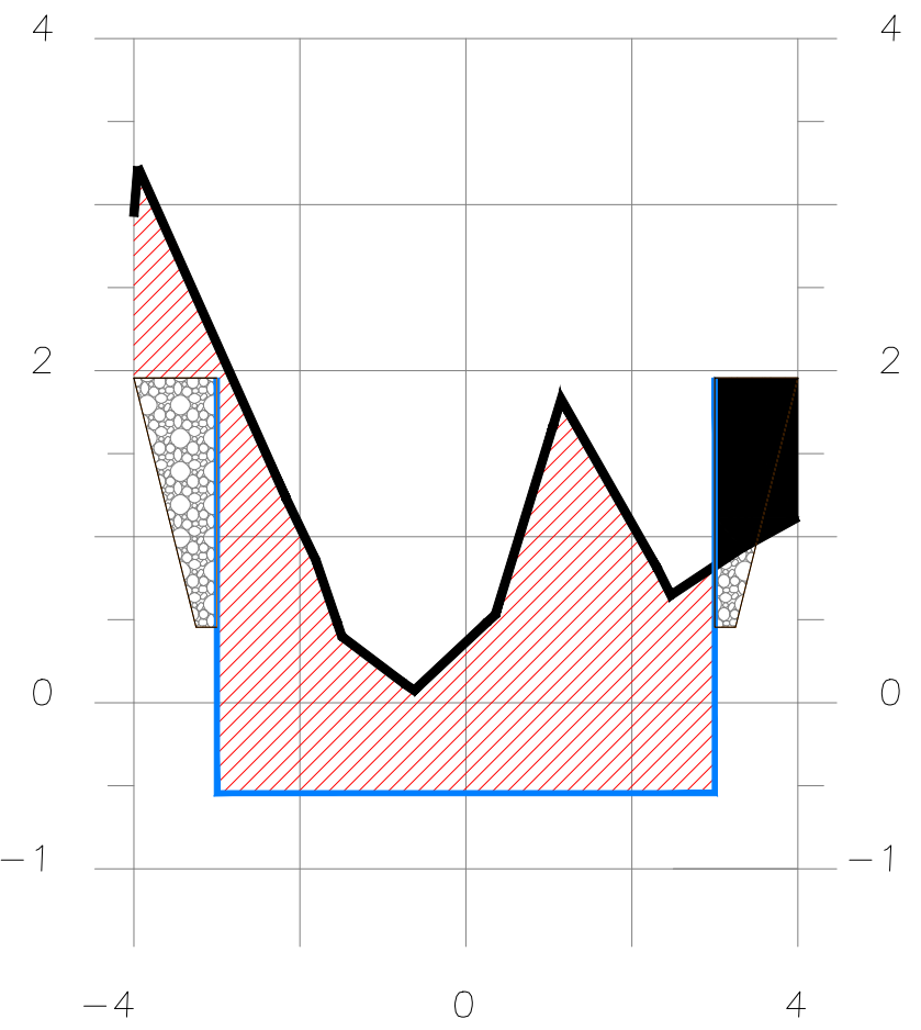
SECCION 3+030
