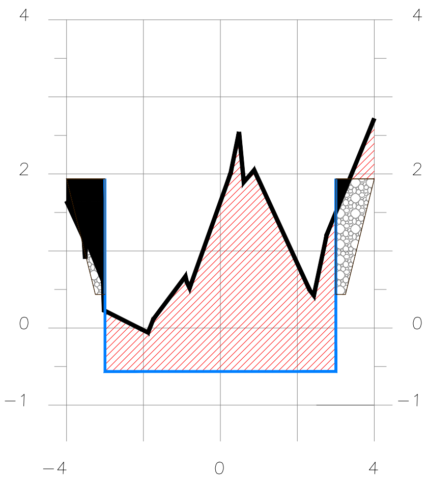
SECCION 3+075
