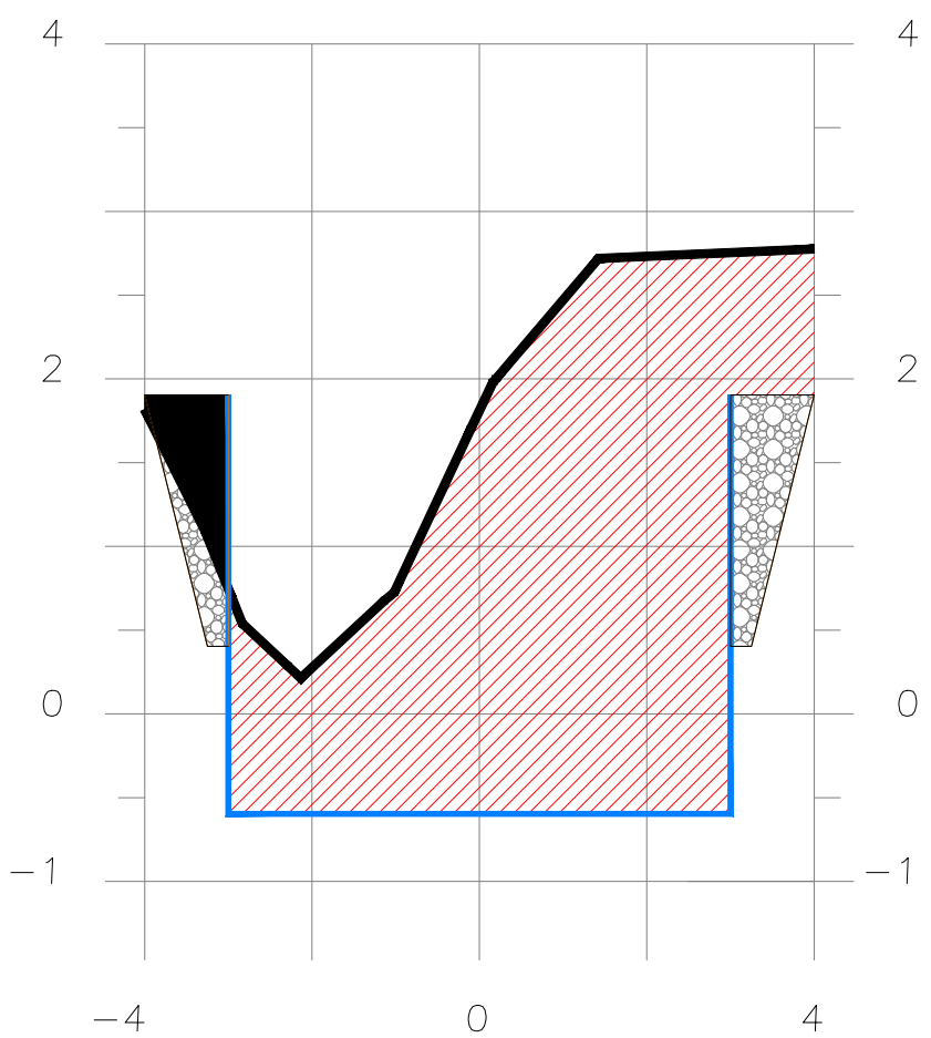
SECCION 3+150
