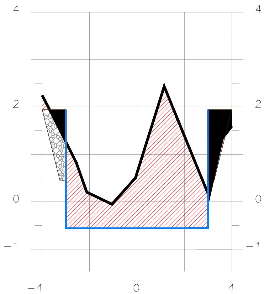
SECCION 3+060
