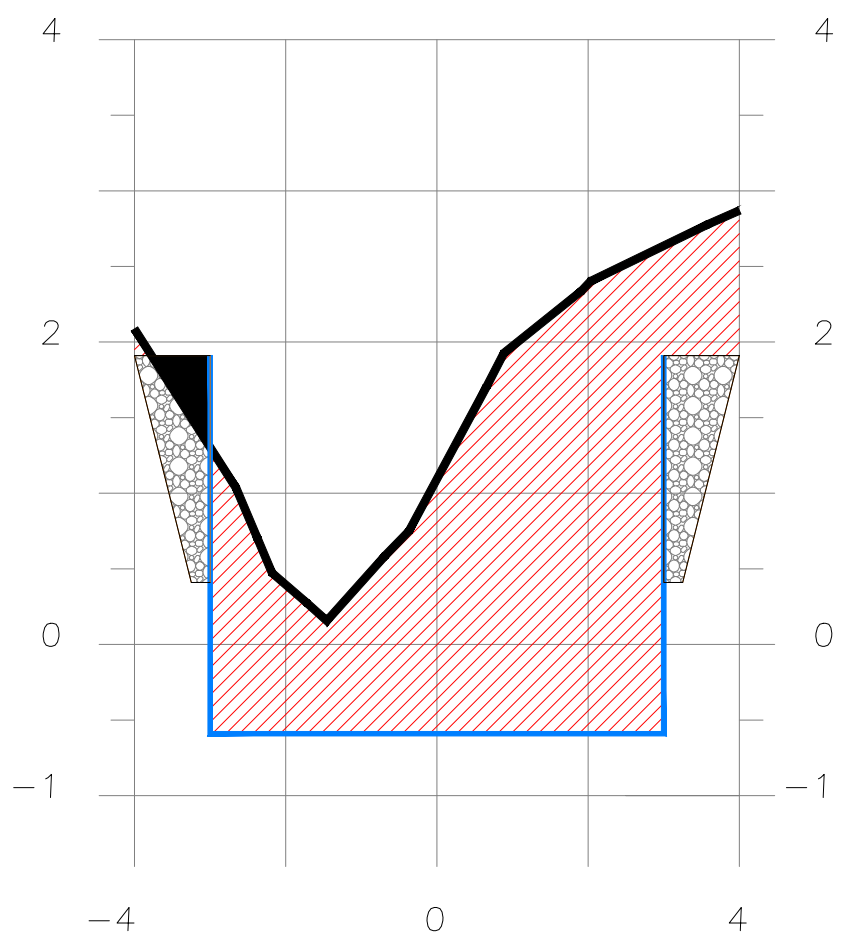
SECCION 3+135
