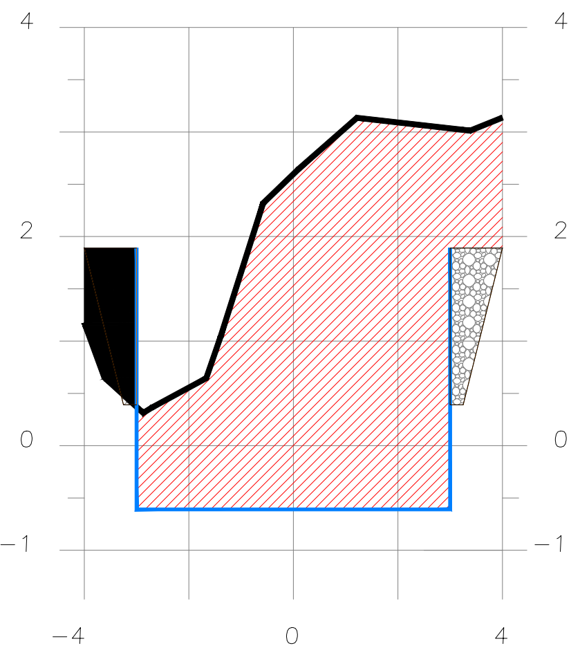
SECCION 3+180
