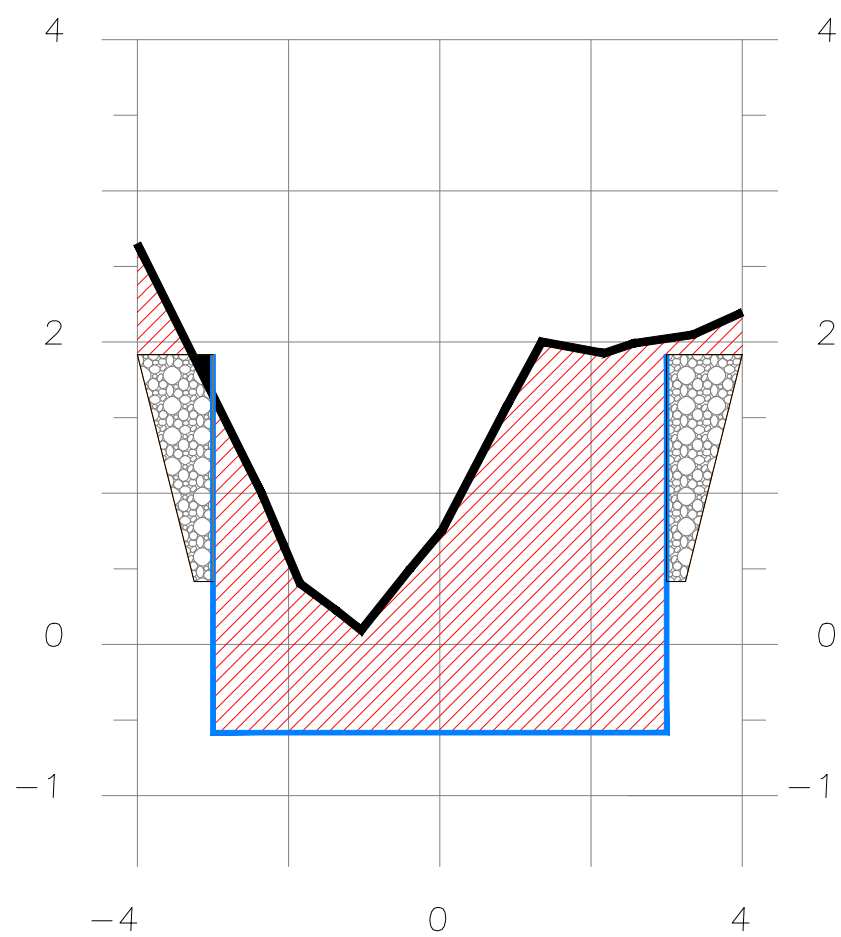
SECCION 3+120
