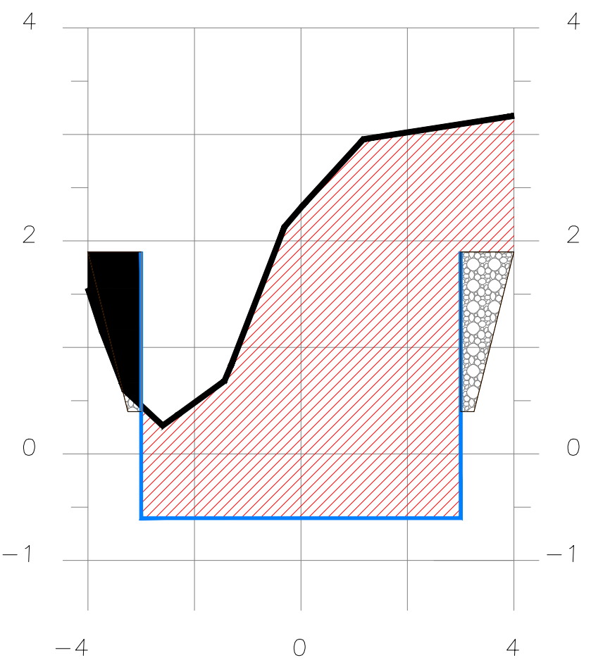
SECCION 3+165
