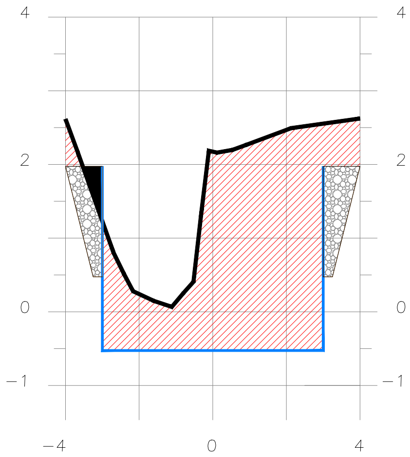
SECCION 2+985
