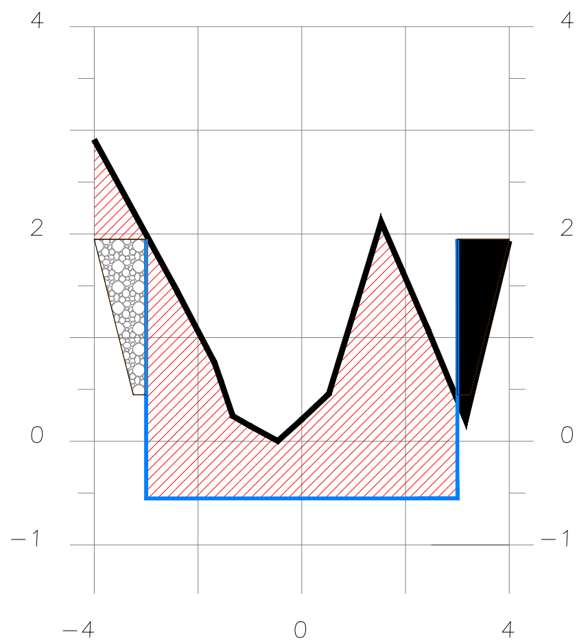
SECCION 3+045
