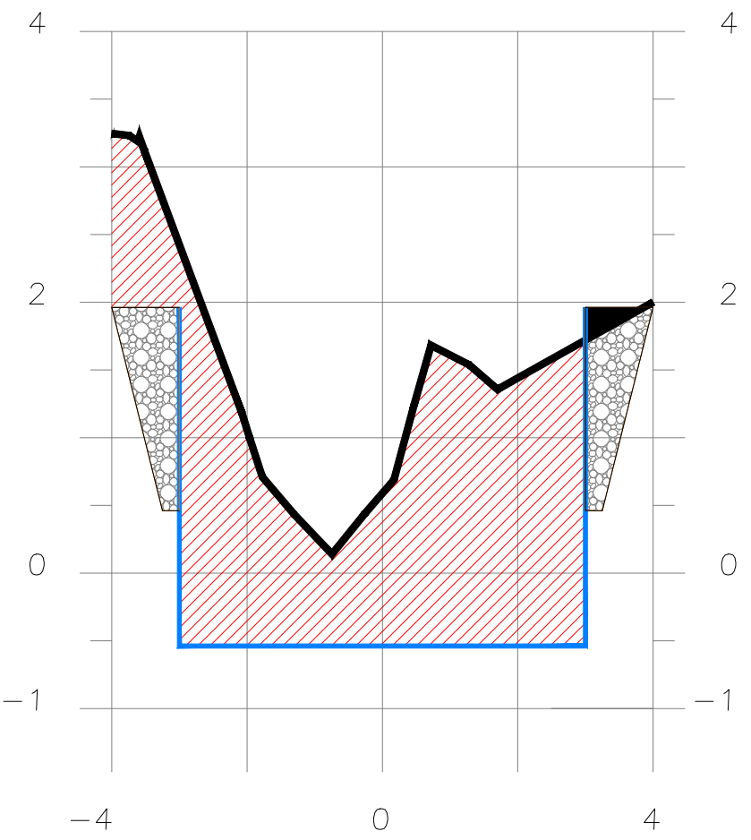
SECCION 3+015
