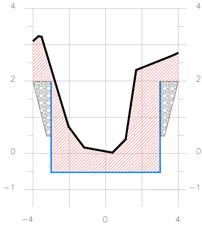
SECCION 2+970
