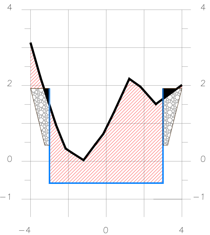
SECCION 3+105
